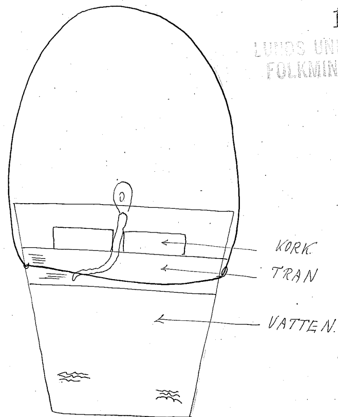
FIG. 2 TRANLAMP AV DRICKSGLAS (ENL. BESKR.)
