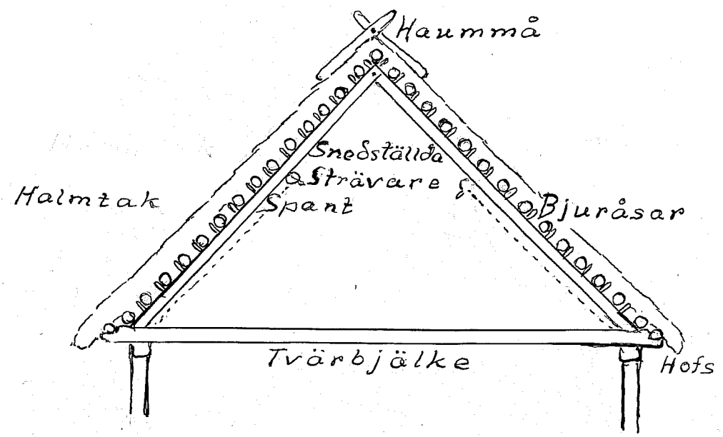
Takstol i ladugård. (Omkring 1850.)
