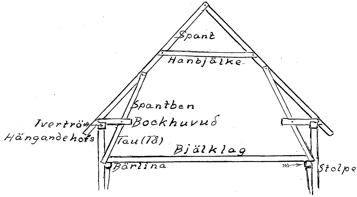
Takstol i lad och höslinne. (1870—)
