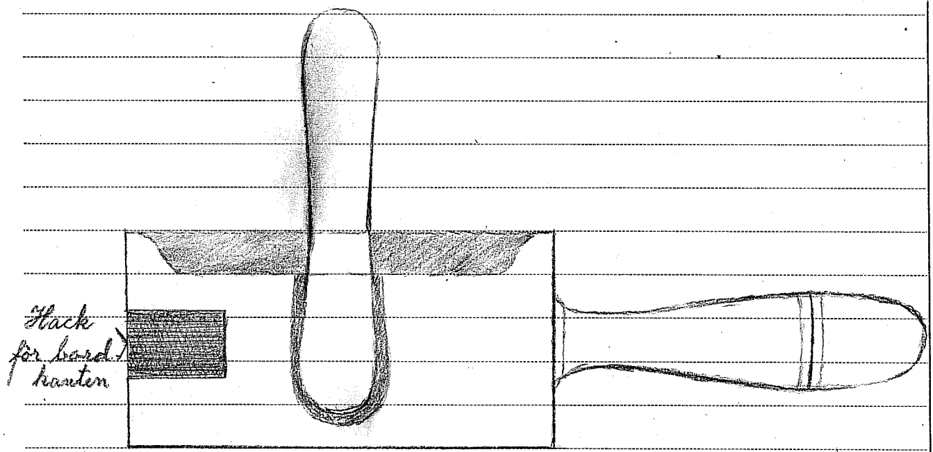
Här en teckning av en hemgjord senapsknäcka, knäckan är gjord av något hått träslag t.x. vitbok eller rödbok rönn eller lönn
